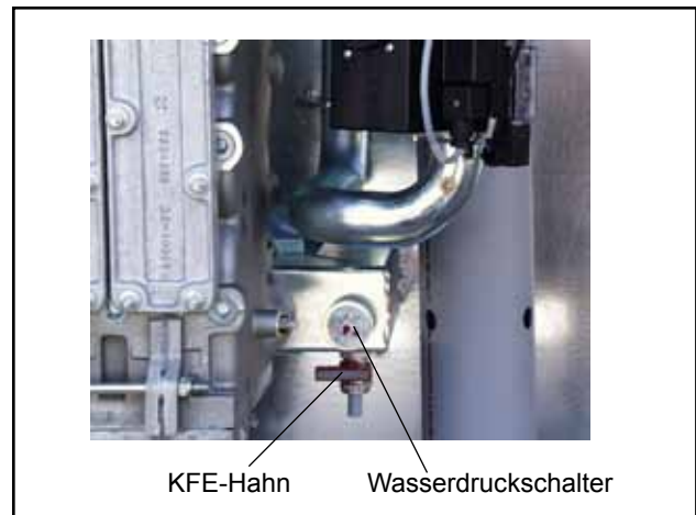
Bild: (KFE-Hahn)
