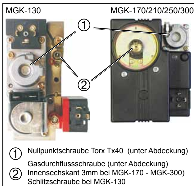
Bild: Gaskombiventil
