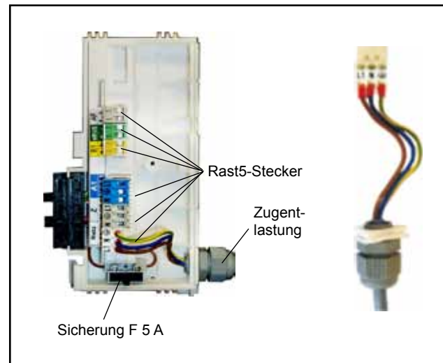
Bild: Anschlusskasten
