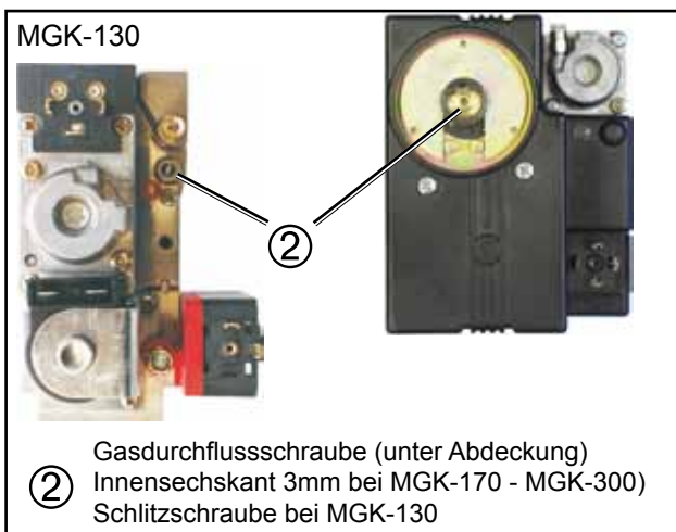
Bild: Gaskombiventil
