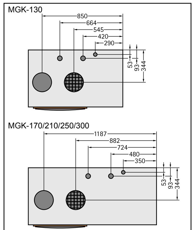
Bild: Anschlussmaße
