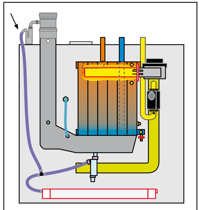
Bild: Kondensatschlauch
