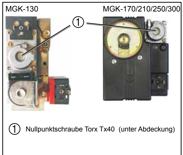
Bild: Gaskombiventil
