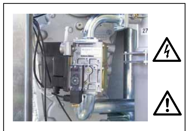
Bild: Gaskombiventil MGK-170/210/250/300 Gefahr durch elektrische Spannung Gefahr von Vergiftung und Explosion durch auströmendes Gas
