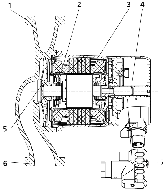
Abb. 2: Schnittbild Pumpe
