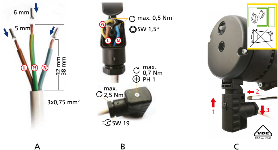
Abb. 7: Netzanschluss
