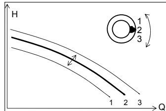
Abb. 3: Einstellung Stellerbetrieb
