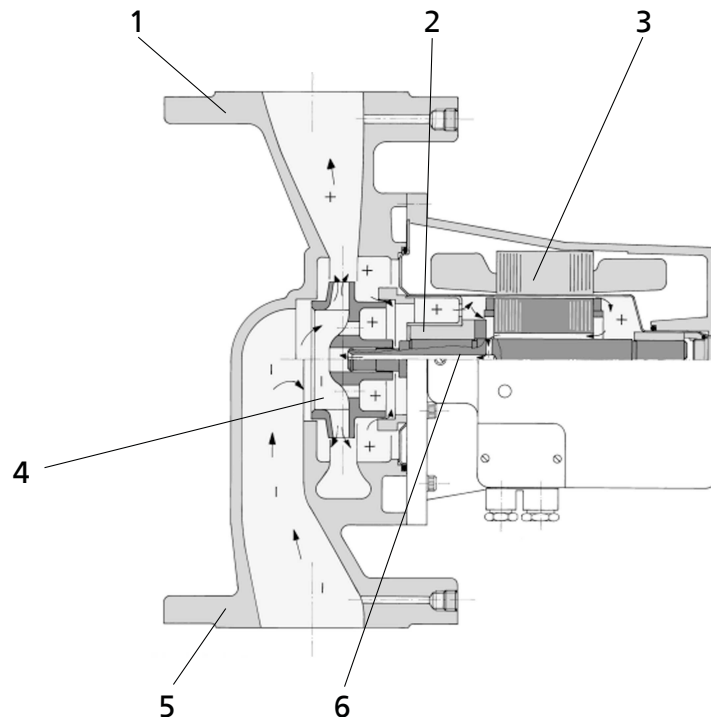
Abb. 2: Schnittbild Pumpe
