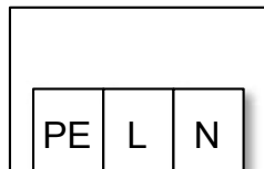
Abb. 4: Anschlussplan Einphasen-Wechselstrom
