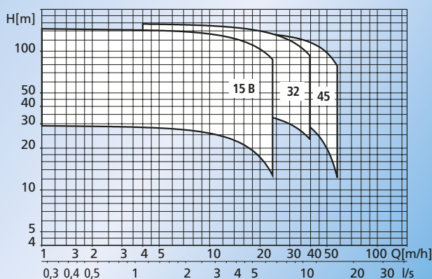
Kennlinien
